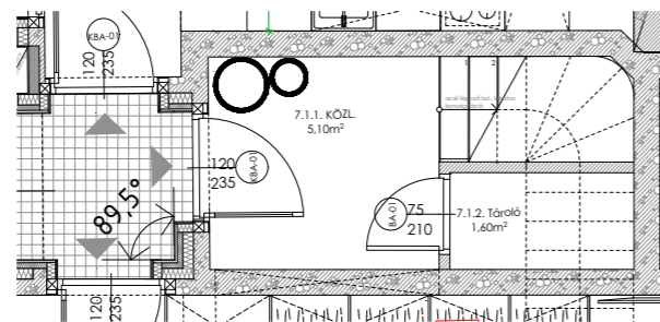
▲ Alsó szint
