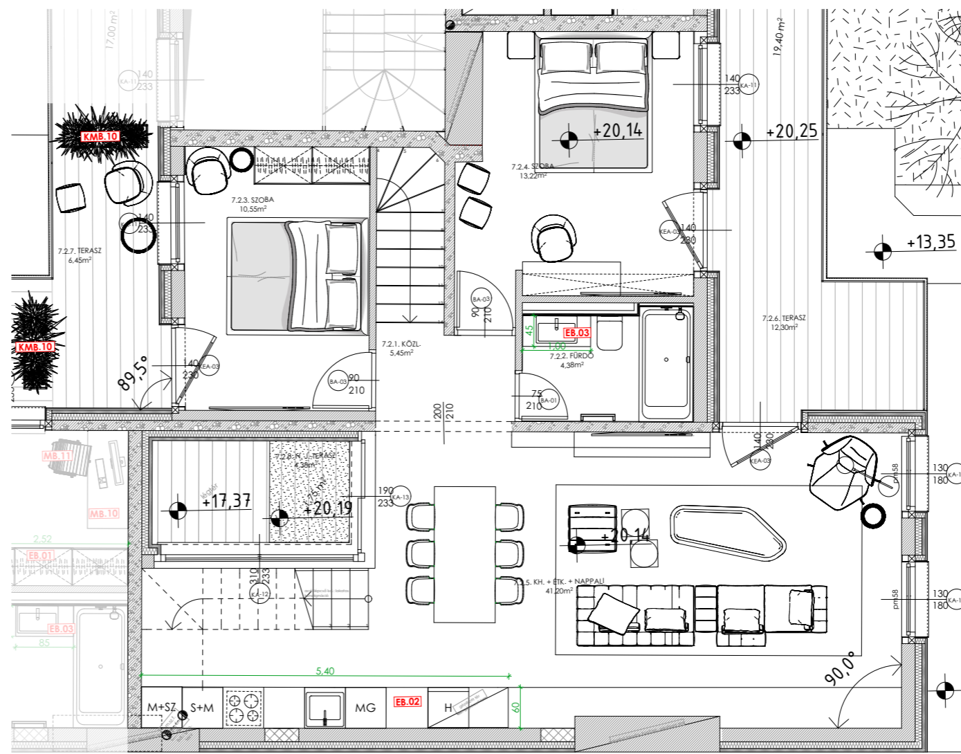
▲ Felső szint
